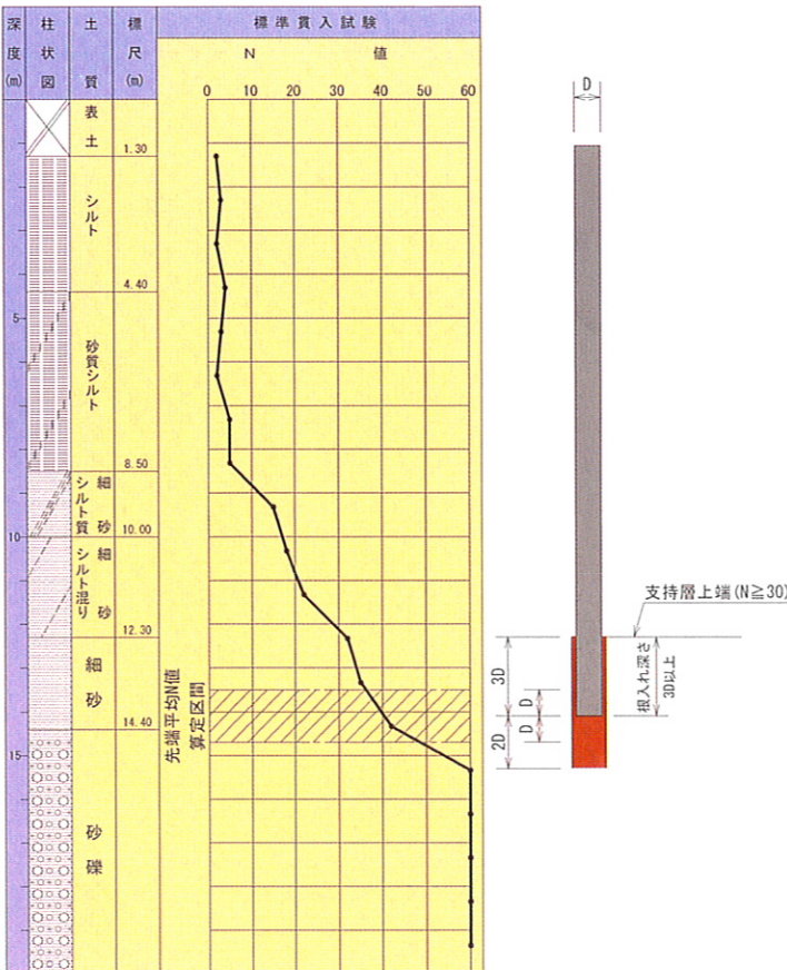
【ストレート杭を用いたプレボーリング拡大根固め工法の支持力係数 \alpha 】
